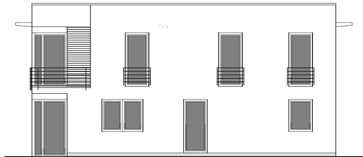
Nord-Ansicht
